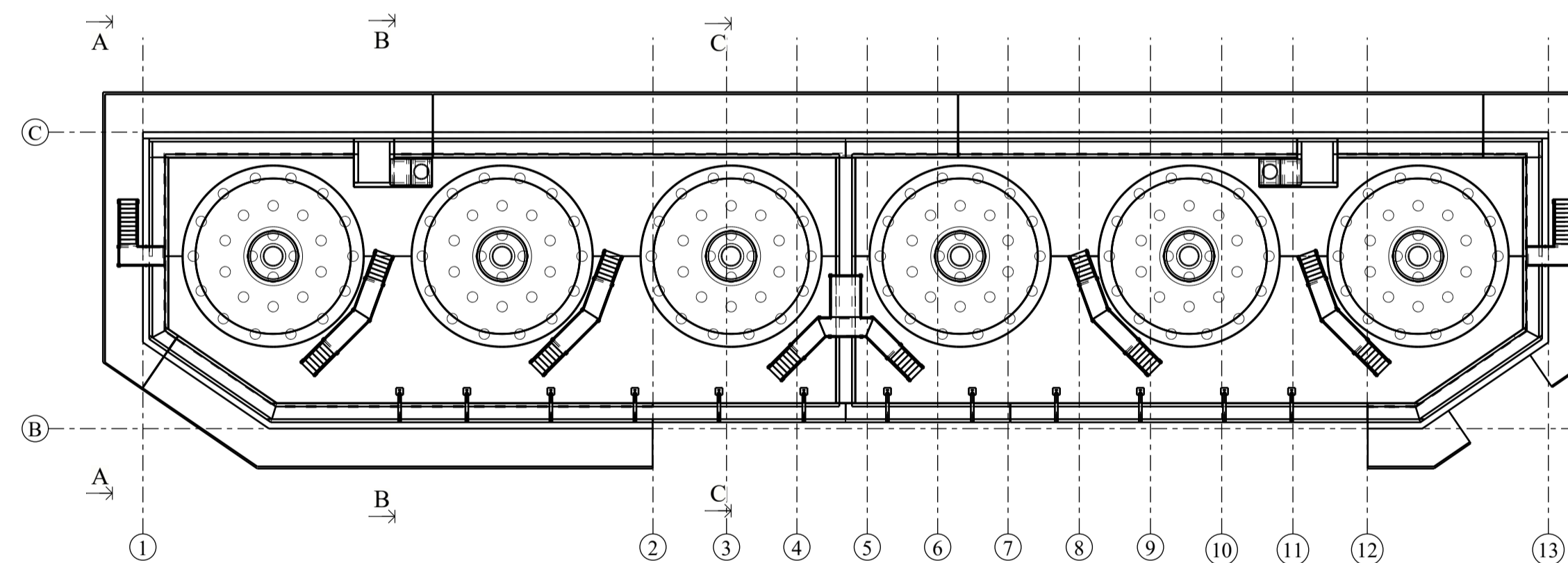
Konstruktivų planas M 1:250
