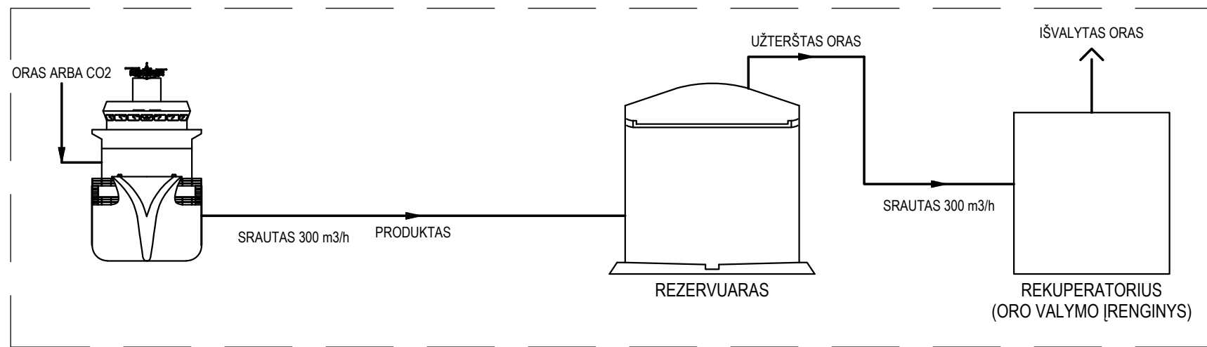
5. LAIVAS → REZERVUARAS
