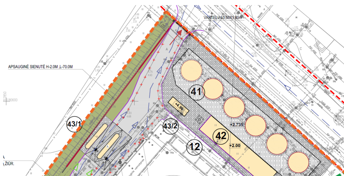
2.9.11 pav. Projektuojama apsauginė sienutė šalia sklypo ribos su AB „Klaipėdos nafta“.
