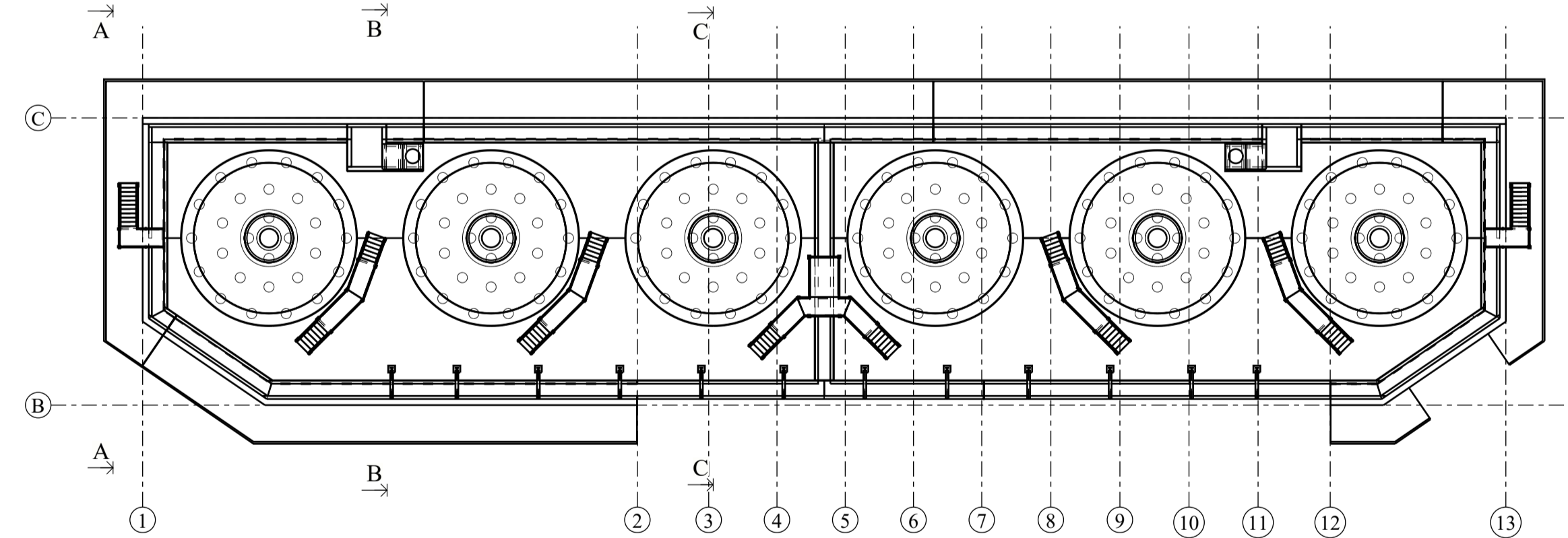
Konstruktivų planas M 1:250
