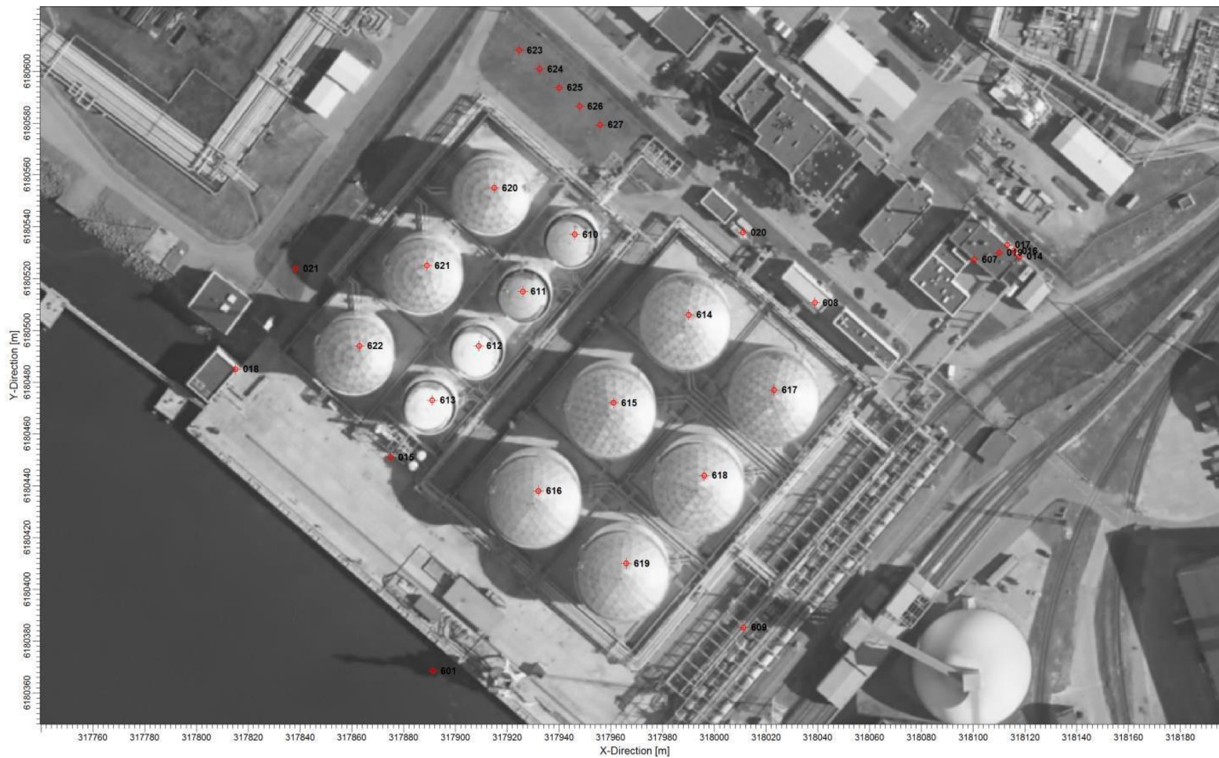
1 pav. Oro taršos šaltinių išsidėstymo schema
