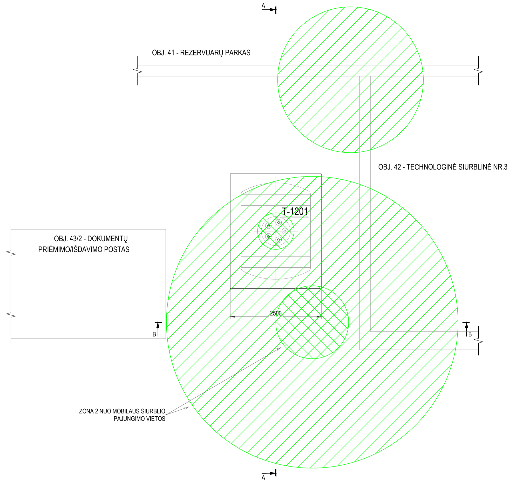
DRENAŽINĖS TALPOS PLANAS DRAIN VESSEL PLAN M 1:50
