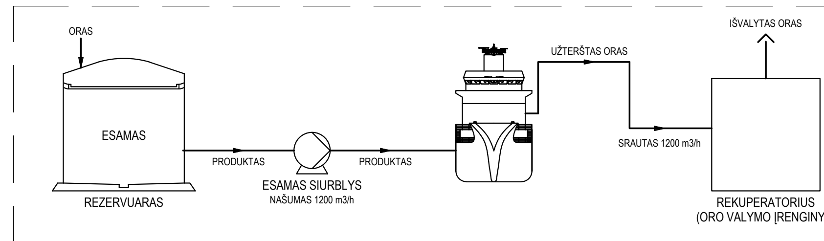
7. REZERVUARAS → LAIVAS
