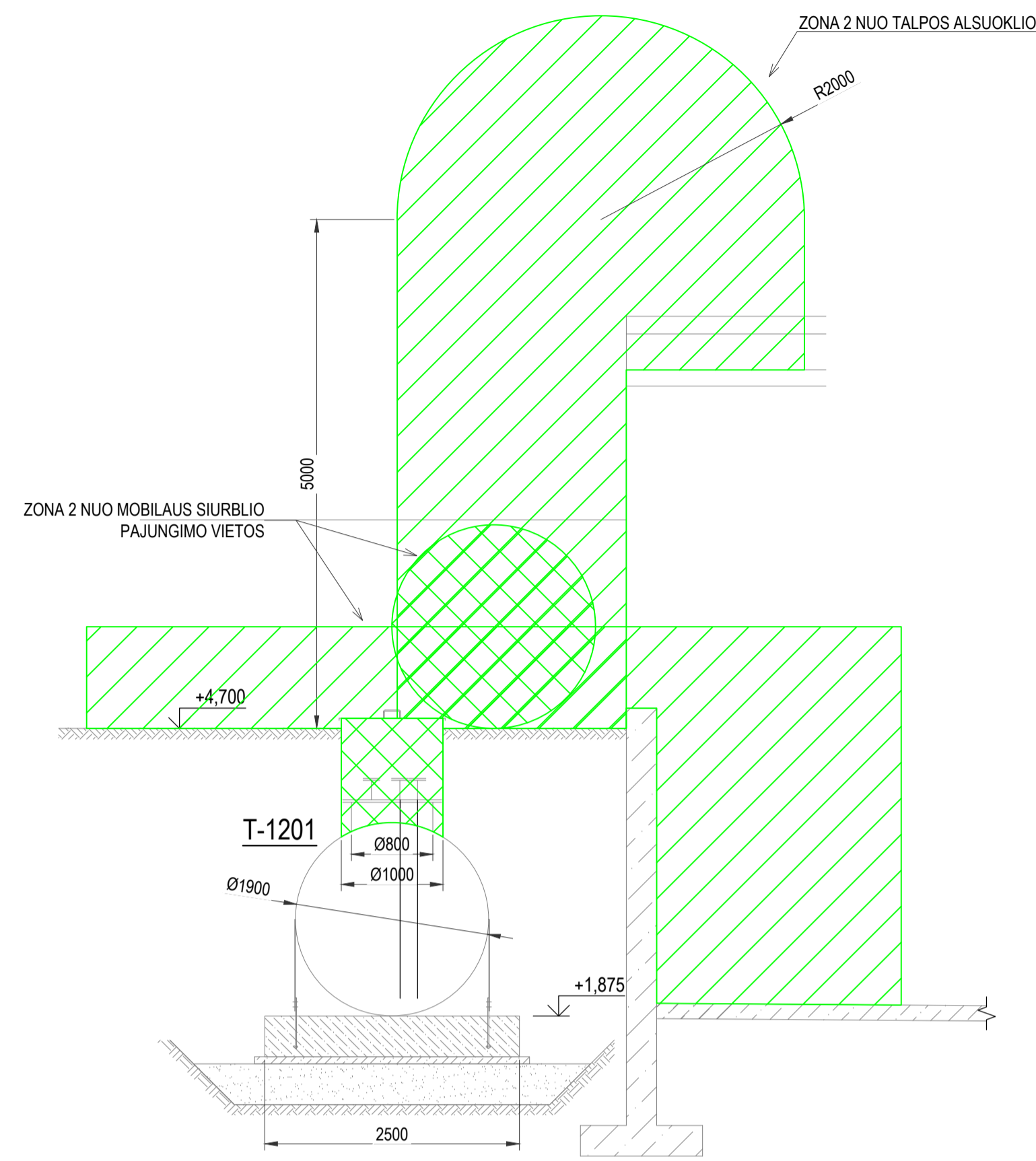
PJŪVIS B-B SECTION B-B M 1:50
