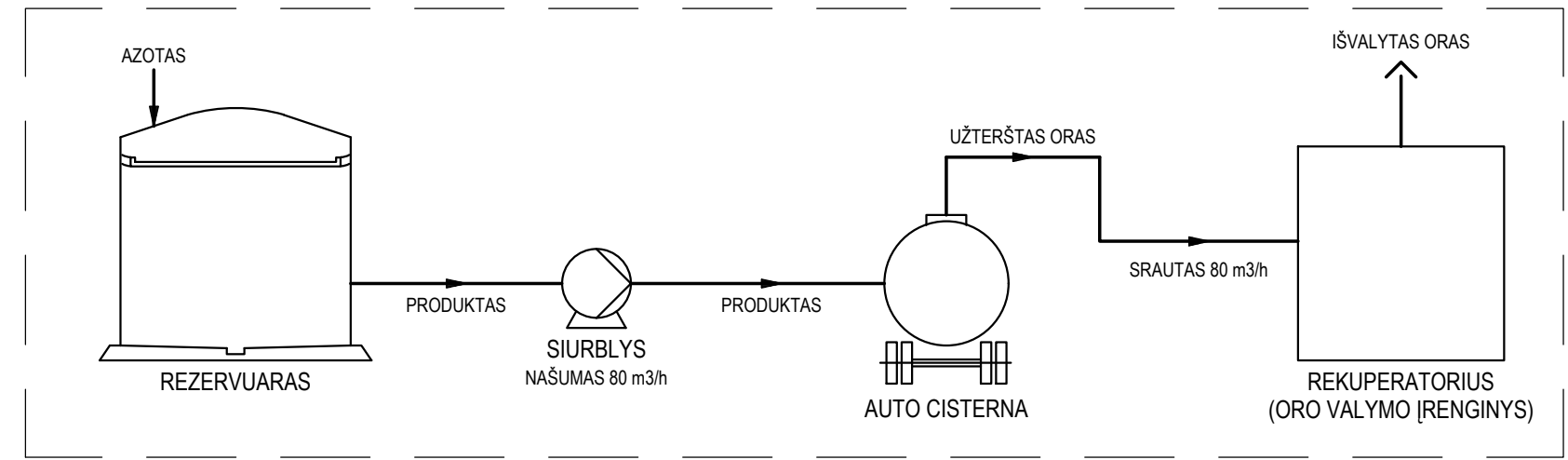
2. REZERVUARAS → AUTO CISTERNA
