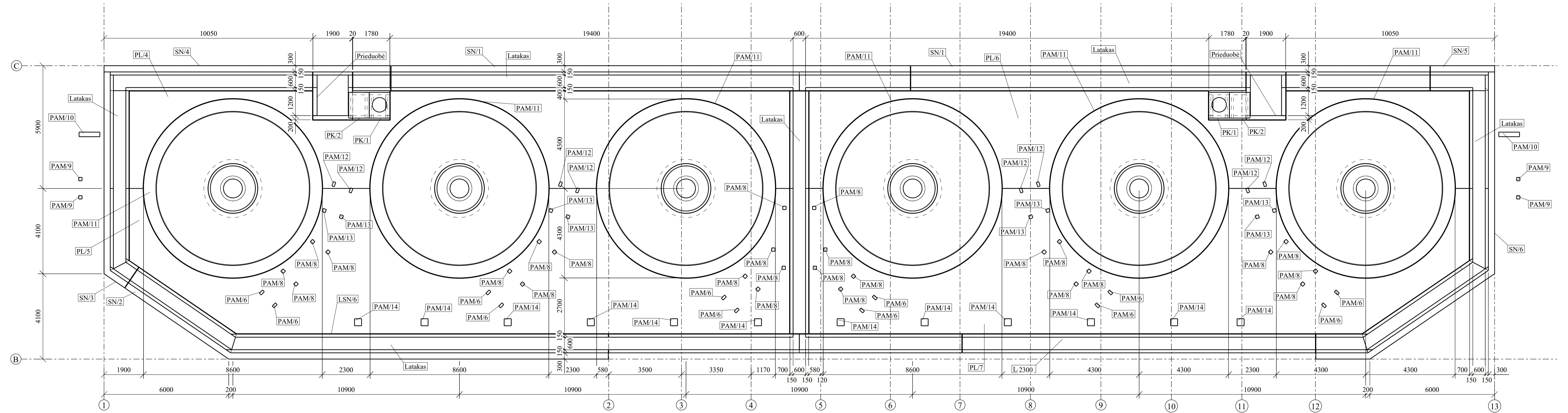
Grindų, latačių ir pamatų planas M 1:100
