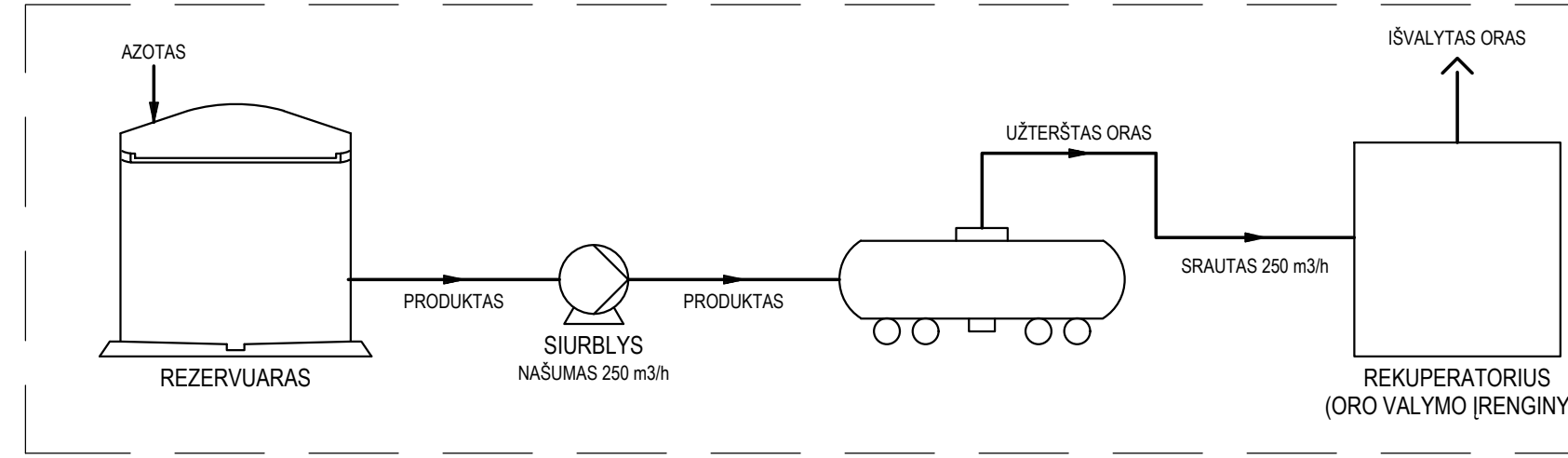
4. REZERVUARAS → GELEŽINKELIO CISTERNOS
