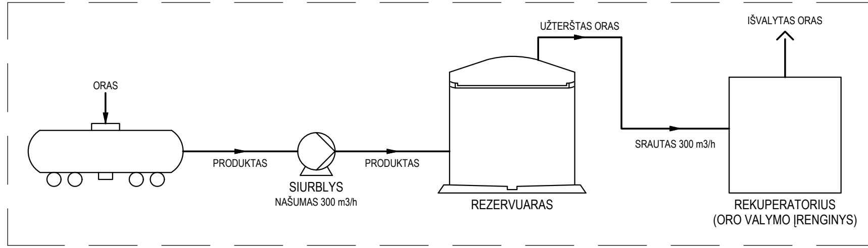
3. GELEŽINKELIO CISTERNOS → REZERVUARAS
