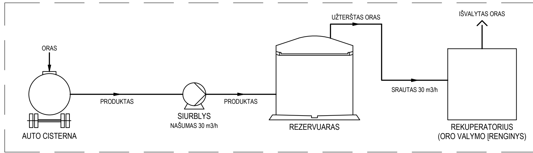
1. AUTO CISTERNA → REZERVUARAS
