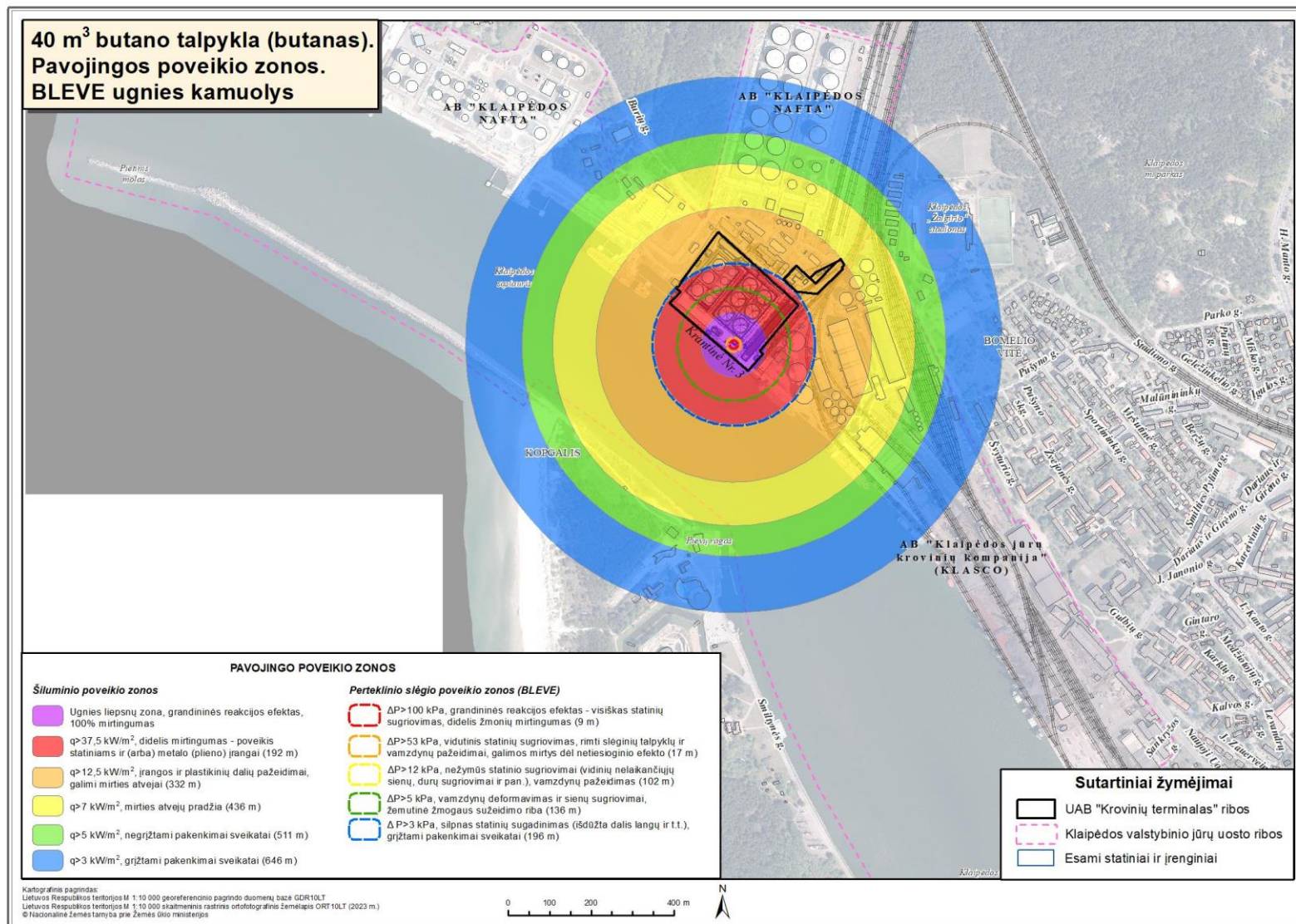
4.1.1 pav. 40 m 3 butano talpyklos BLEVE ugnies kamuolio pavoingos poveikio zonos (įvykio tikimybė 6,93E-08).
