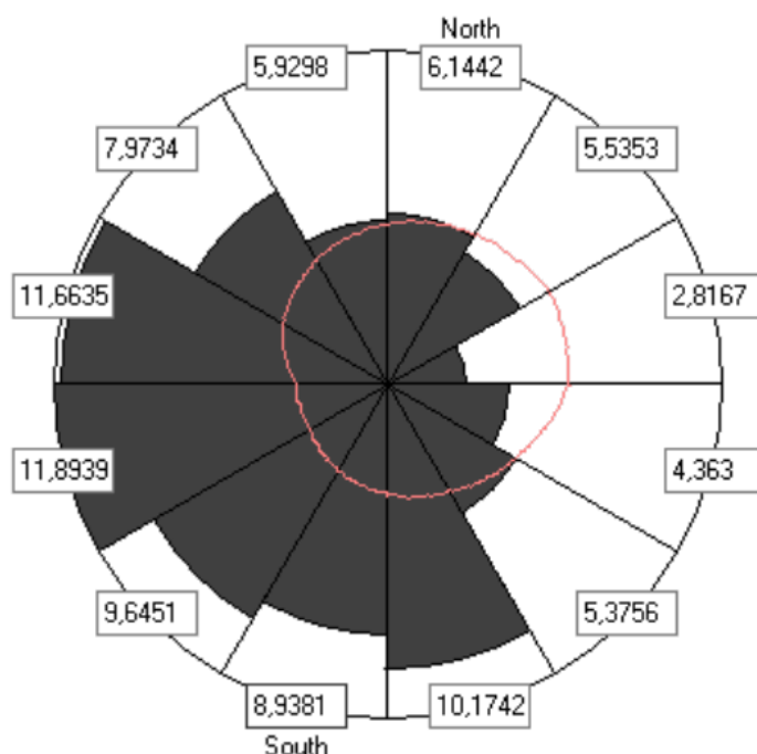
Pav. 7. Kauno miesto vėjų rožė, sudaryta CadnaA programoje
