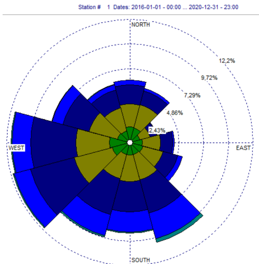
Pav. 11. Kauno hidrometeorologinės stoties vėjų rožė (kryptis – pučia iš)
